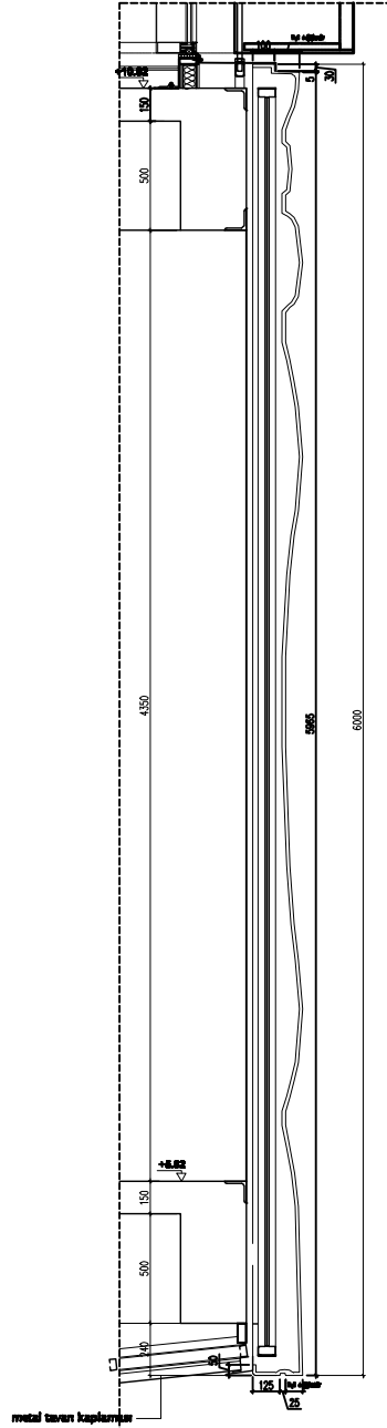
KESİT
